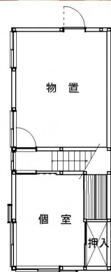
地階平面図
