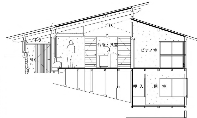
断面
