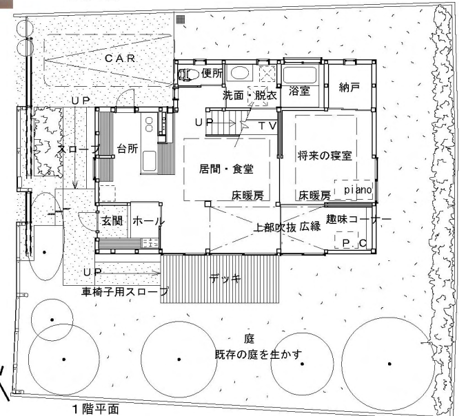
1階平面
