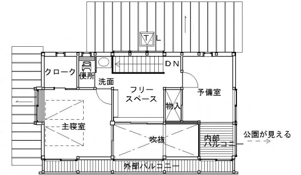
2階平面
