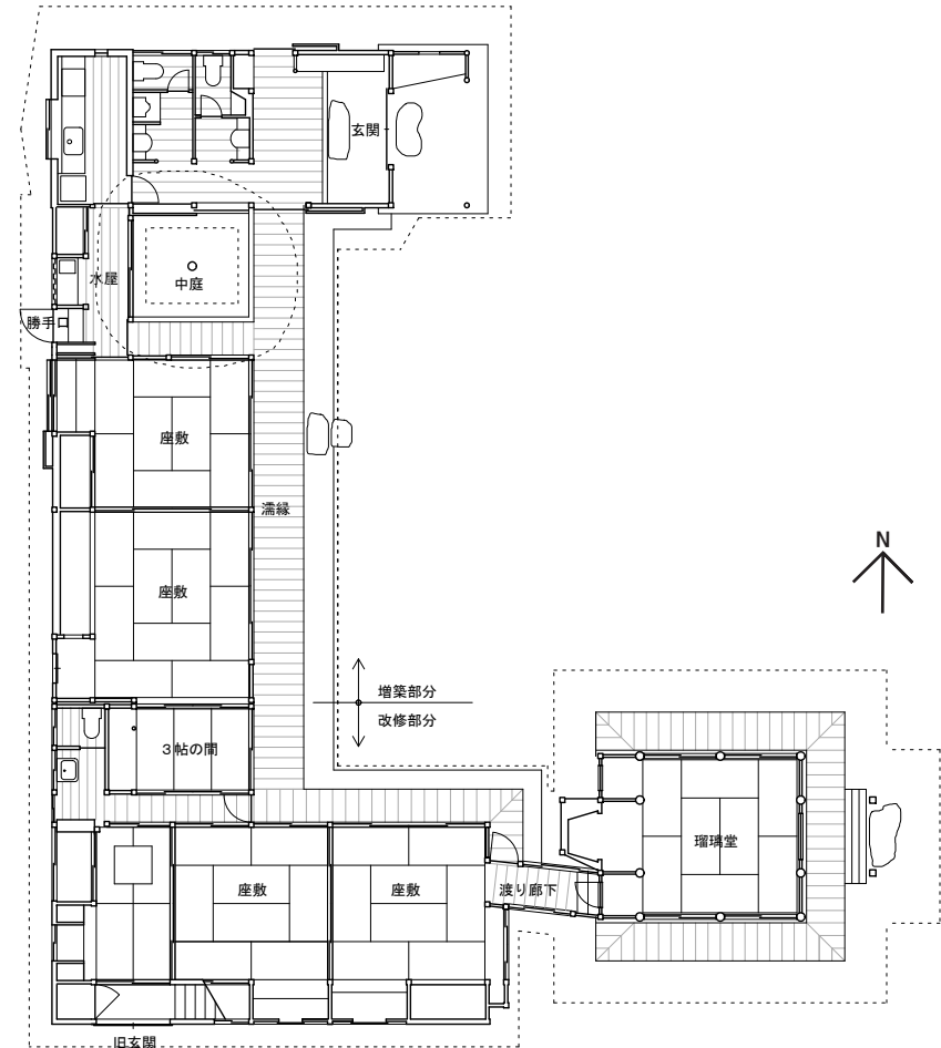
平面図
